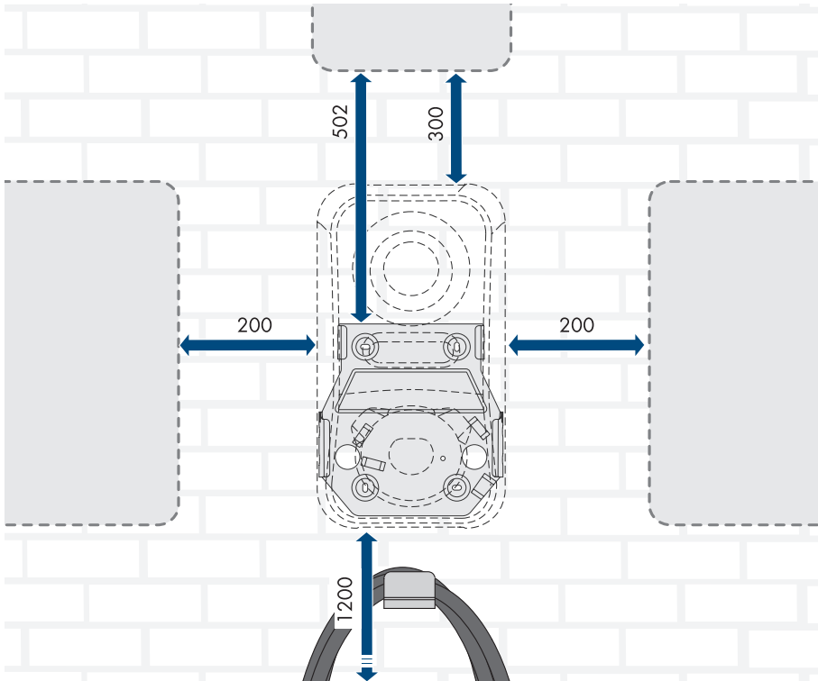
Abbildung 9: Empfohlene Abstände
