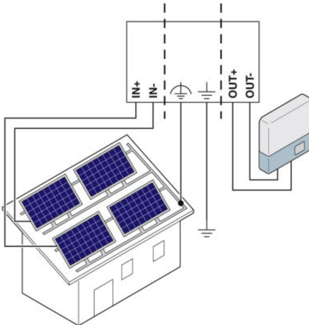
Anschlusszeichnung
